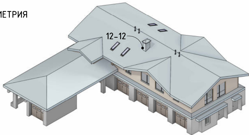
АКСОНОМЕТРИЯ УЗЛА 12-12 (СЕЧЕНИЕ)
