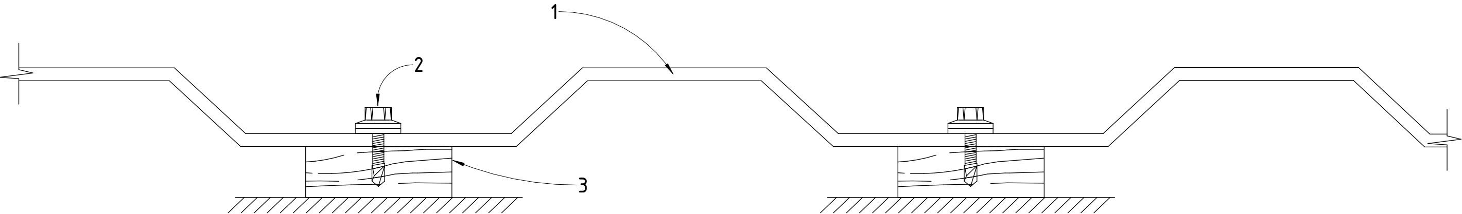
1. Композитный профилированный лист С - 20 "ETIZ" (ссылка) 2. Саморез кровельный с компенсационной прокладкой (ссылка)" 3. Доска конструктивная. Обрешетка кровли
